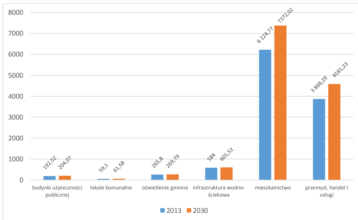
Wykres 12 Zmiana zużycia energii elektrycznej w latach 2013-2030
