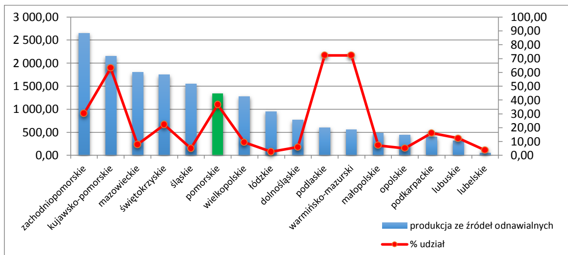
Wykres 14 Wartość produkcji energii ze źródeł odnawialnych w podziale na województwa w 2013 roku
